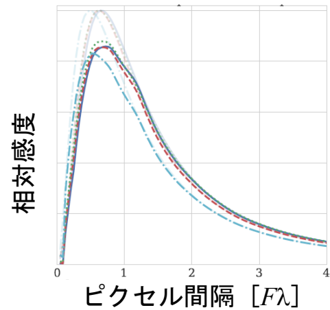
図 2: ピクセル間隔と感度の関係。淡色の線は強度相関を考慮しなかった場合。
