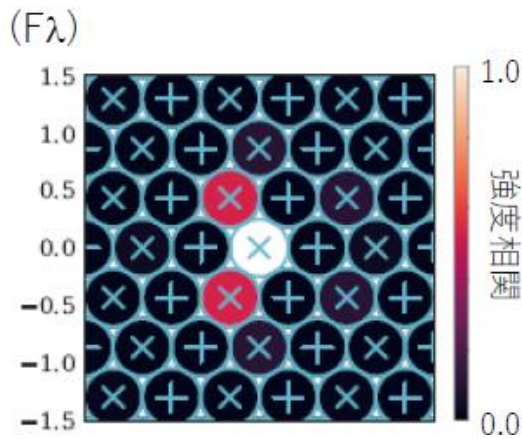
図 1: ピクセル間の相関パターンの例。色で中央のピクセルとの相関を表す。
