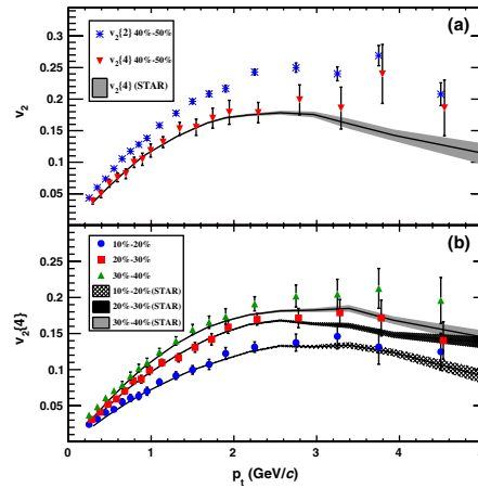
図 1 LHC-ALICE 実験で初めて観測された方位角異方性 v_2 の横運動量依存性。横運動量が 3 GeV/c において RHIC 実験と良い一致を示すことがわかった(論文⑧)。
