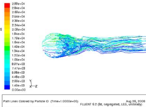
図 4 サッカーボール回りのパスライン。
