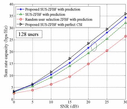
図1 通信路予測を用いた MU-MIMO の通信路容量と特性
