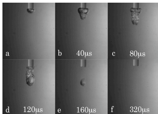
図3 平坦型チップによる気泡パターン
