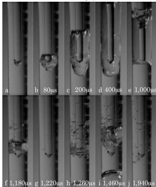
図4 模擬根管内での気泡パターン
