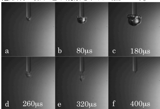
図2 円錐型チップによる気泡パターン
