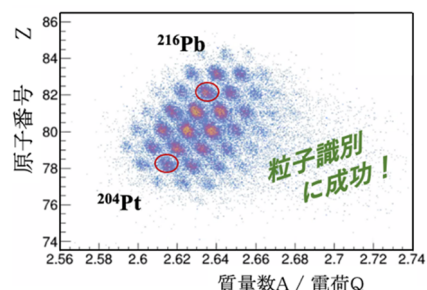
図 3 : N=126 領域の崩壊測定実験
