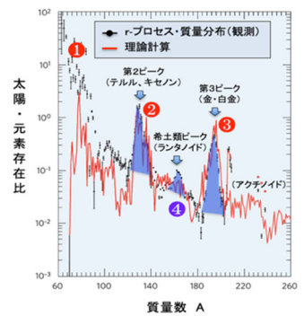
図1：太陽系 r-プロセス成分
