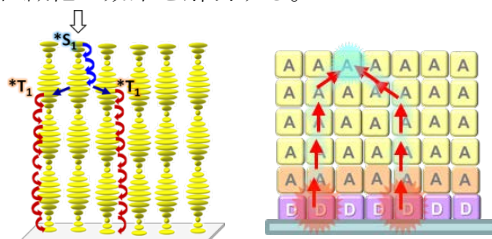
図2 (a) キラル組織化 SF, (b) TTA-UC 増強システム
