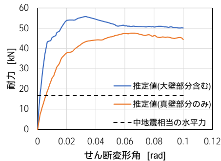
図9 対象建物の荷重変形関係
