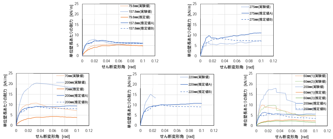
図7 推定値と実験値の荷重変形関係
