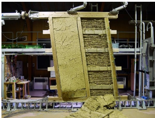
写真 1 試験体 2 最大変形時 (1/8.4rad)
