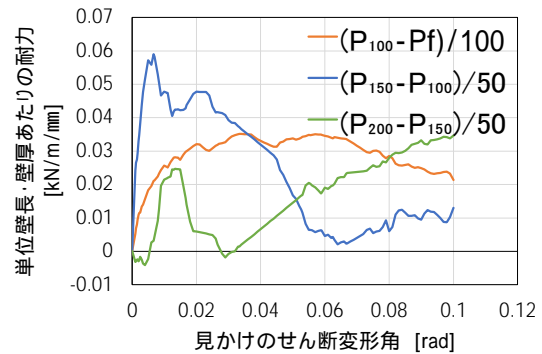
図6 壁厚さ 1mm あたりの耐力
