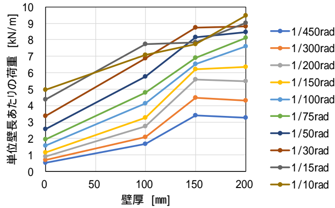
図4 耐力と壁厚の関係
