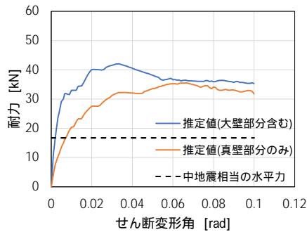
図9 対象建物の荷重変形関係
