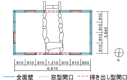
図8 対象建物平面図
