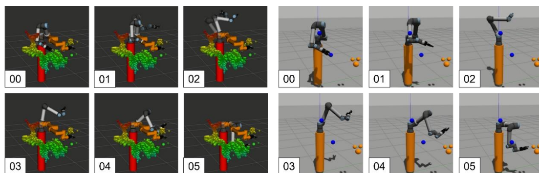
(a) ロボットアーム周囲の障害物認識 (b) 障害物回避による果実収穫
