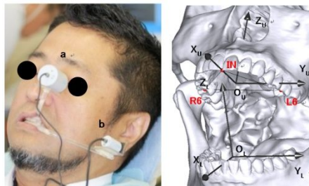
一対の三軸コイルセンサ a: 一次コイル b: 二次コイル
