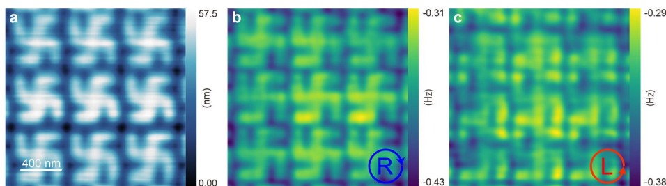
図3 円型キラリティな金ナノ構造体の円偏光光誘起力顕微鏡観測。a)凹凸像。b, c)右回りおよび左回り円偏光照射時の PiFM 像。
