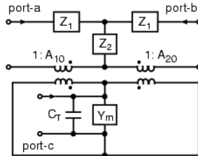
図1：楕形電極の等価回路モデル
