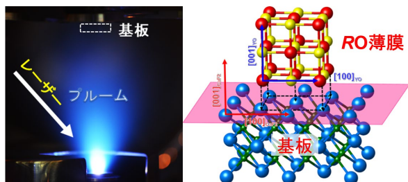
図 1 紫外レーザー (左) で合成できる岩塩構造希土類単酸化物の結晶構造 (右)
