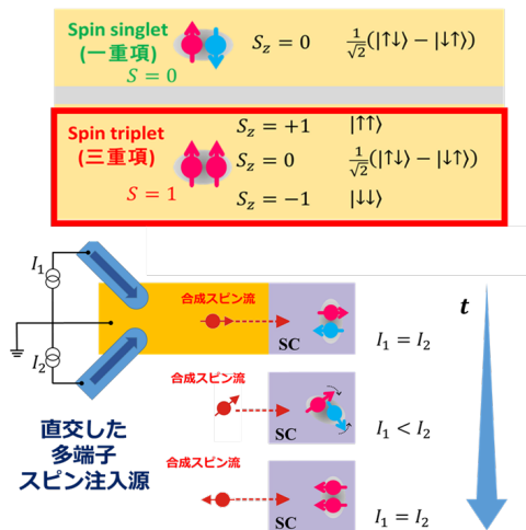
図1. 回転スピン流によるスピントリプレット・クーパ対の形成
