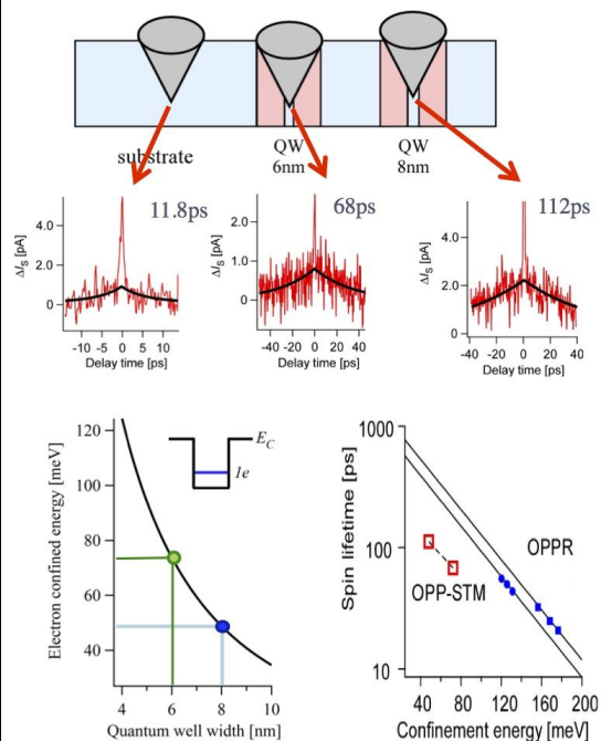
図7 GaAs/AlGaAs量子井戸(井戸幅6nm, 8nm)中に、円偏光により励起・配向されたスピンの乱れていく緩和過程の時間分解測定スペクトル(上段)と、量子井戸幅と閉じ込めエネルギーの関係(下段左)、得られた寿命と閉じ込めエネルギーの関係(下段右)。OPPRの結果(青丸)は、多重量子井戸の構造に対して行われた平均的な情報を与える光学測定の結果。Nature Nanotechnology 9, 588 (2014), 文献リスト4。
