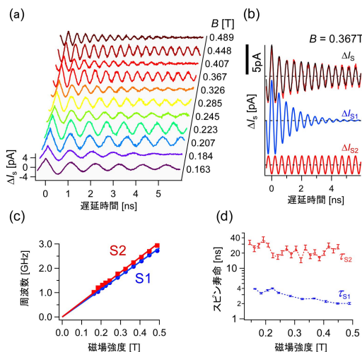
図9 磁場中でのスピン歳差運動の時間分解STM測定の結果。(a) スペクトルの磁場依存性。(b) フィッティングにより得られた二つの成分。(c) 二つの成分のラーモア振動数の磁場依存性。(d) スピン寿命の磁場依存性 Nature Nanotechnology 9, 588 (2014), 文献リスト4。
