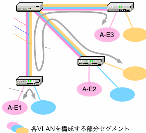
図 1 仮想化ネットワークの例
