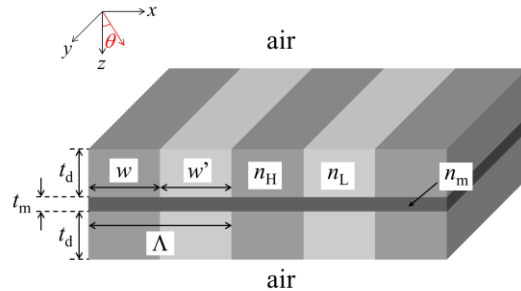
図 1 金属 (Ag) 薄膜と誘電体グレーティングで構成される偏波分離器
