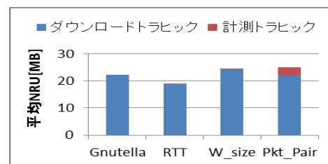
図 4 平均 NRU
