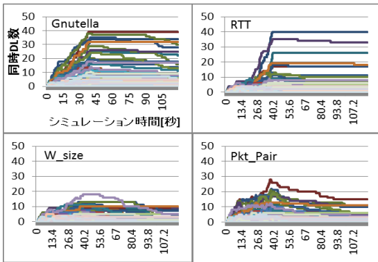
図 5 同時 DL 数
