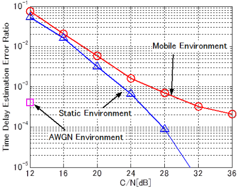
図 8 時間遅延量の判定誤り率特性
