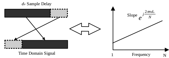
図 2 時間遅延と位相回転量の関係
