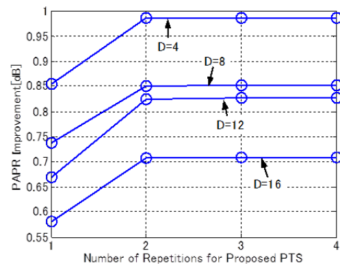
図6 従来方式からのPAPR特性の改善量
