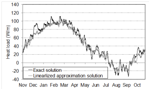
図5 地下室の貫流負荷比較 (GL-2.0m)
