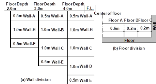
図4 算出した線形近似単位応答の部位
