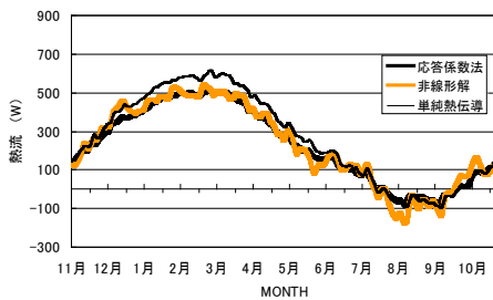
図2 基準気象条件下(東京)における地下室表面熱流の比較
