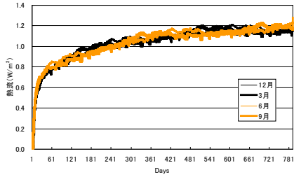
図1 外気温変化に対する地下室内表面熱流の単位応答
