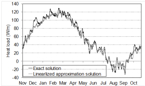
図7 地下室の貫流負荷比較 (GL-3.0m)
