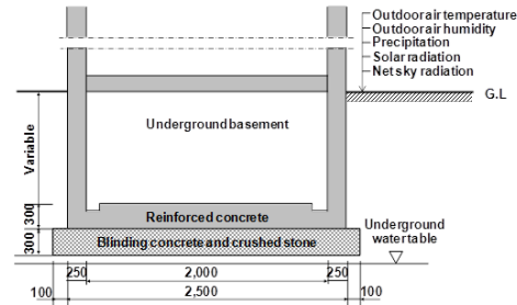
図3 対象とした一般形状の地下構造物
