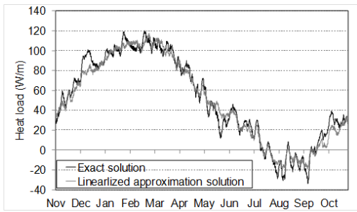
図6 地下室の貫流負荷比較 (GL-3.0m)
