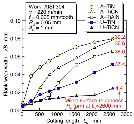
図4 切削距離と逃げ面摩耗幅の関係
