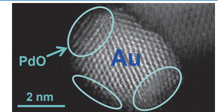
図2 酸化パラジウム(PdO)-on-金(Au)ナノ粒子構造の創製。異種金属界面で種々基質の活性化可能。
