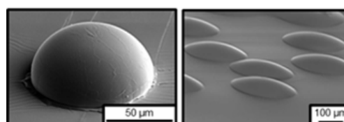
マイクロレンズのSEM像
