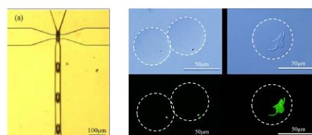
ゲルドロプレット内で培養された細菌
