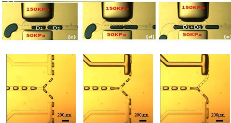
ドロップレットの融合と分割
