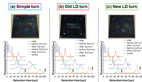
LC CHIP によるたんぱく質の分析
