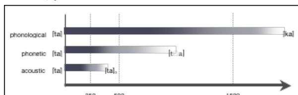
図 2. 音響手がかりのフェードアウト (Pisoni, 1973; Werker & Logan, 1985 に基づく)
