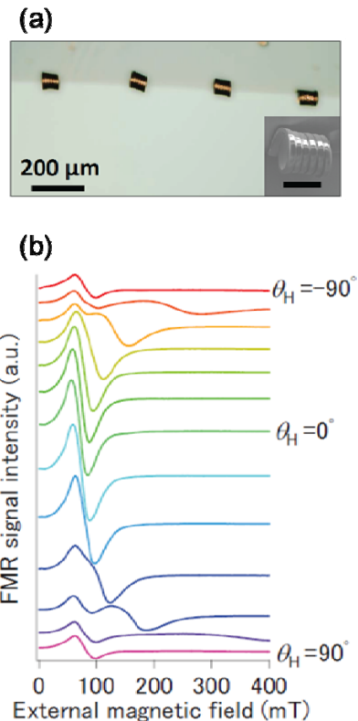
図3 (a)強磁性カイラルメタ分子、(b)角度分解電子スピン共鳴スペクトル
