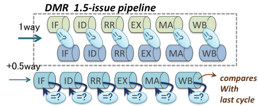
図 4. 1.5-way プロセッサ
