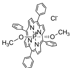
図2 DMP(V)TPPの構造
