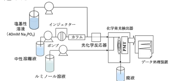
図 1 測定システムの構成
