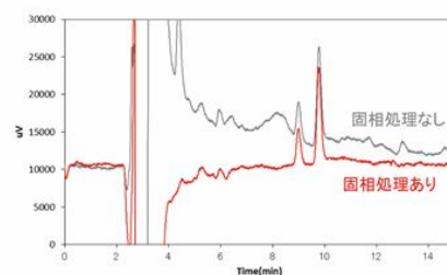
図 3 固相抽出による測定妨害物質除去
