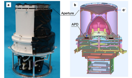
図3 あらせ衛星搭載電子計測器 [Kasahara et al., EPS 2018]
