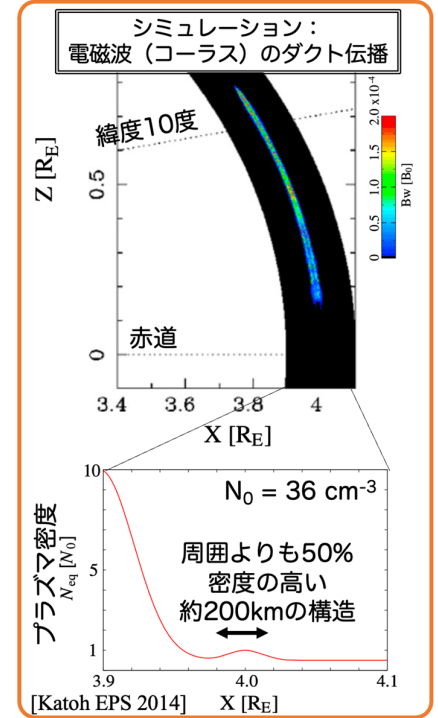
図2 ダクト構造に沿った電磁波の伝搬
