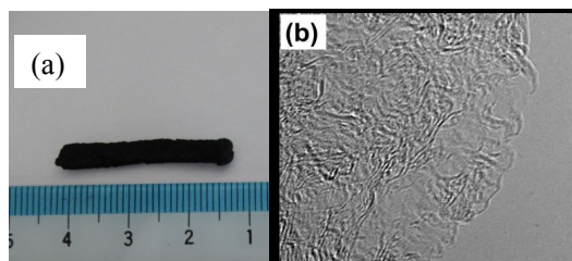
図7. グラフェンモノリス(a)とその透過電子顕微鏡像(b)
