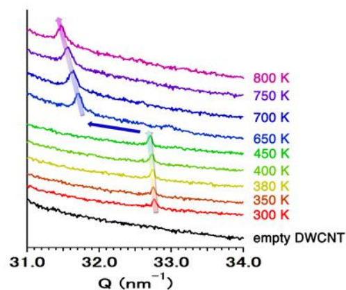
図 2 . 1D 硫黄結晶の X 線回折の温度変化
