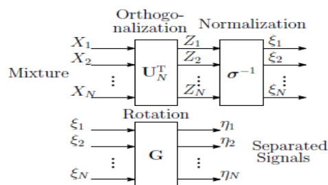
図4 独立成分分析
