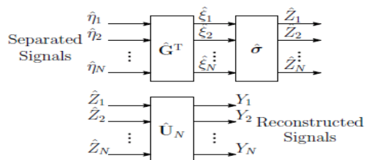
図5 独立成分の再合成
