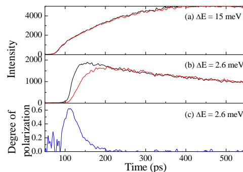
図1. PL 強度と偏極度の時間発展
