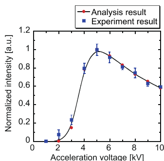
図 4 シミュレーションと実験結果の比較
