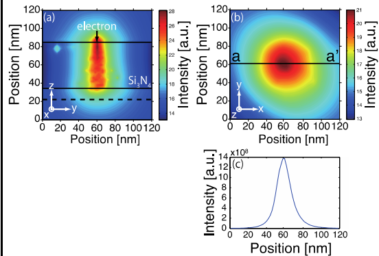
図1 窒化シリコン薄膜に電子線を照射したときに形成される光強度分布の計算結果
