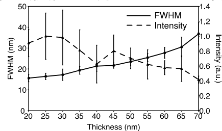
図2 光ナノスポットのサイズ及びその光強度と窒化シリコン薄膜の関係
