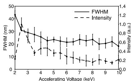
図 3 光ナノスポットのサイズ及びその光強度と入射電子の加速電圧の関係
