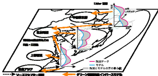
図1 本研究の観測・データ同化の連携の模式図
