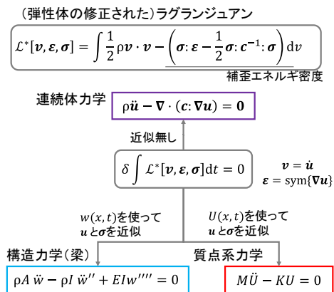
図2. メタモデリングの理論: ラグランジュアンと数理近似
