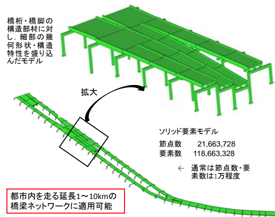
図3. 自動構築された橋梁ネットワークのモデル
