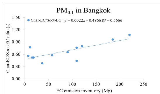
図2 バイオマス燃焼指標(Char-EC/Soot-EC)と元素状炭素(EC)排出インベントリとの関係
