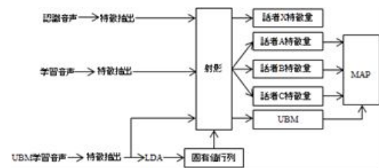
図1 UBM 特徴空間に対する判別分析の適用の流れ
