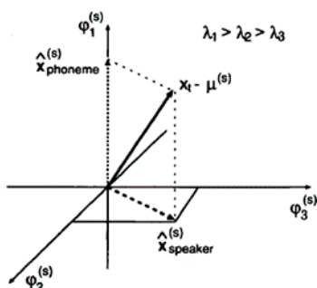
図 2 音韻ベクトルと話者ベクトル
