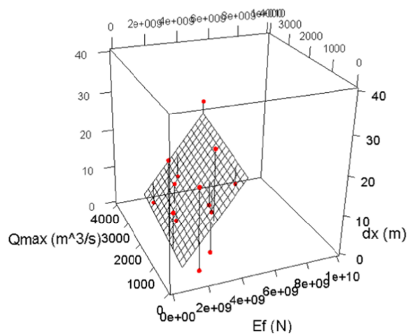
図 8 波浪および流量とテラス斜面部の沖向き移動量の関係
