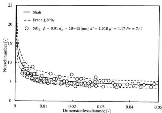
(b)シリカ・ナノ流体の熱伝達
