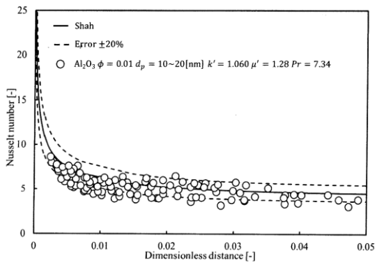
(a)アルミナ・ナノ流体の熱伝達
