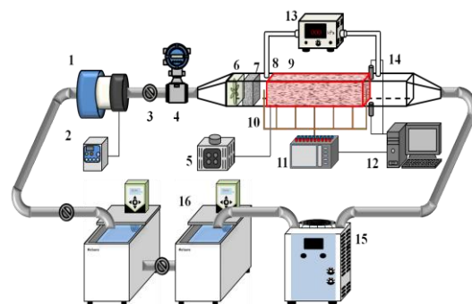
図 2 熱流動実験装置の概略
