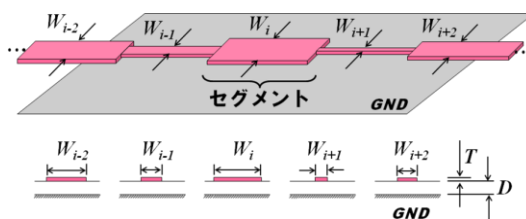
図1 STLの概略
