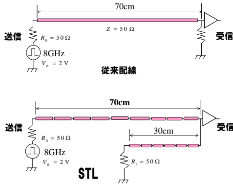
図 9 有損失従来配線と有損失 STL
