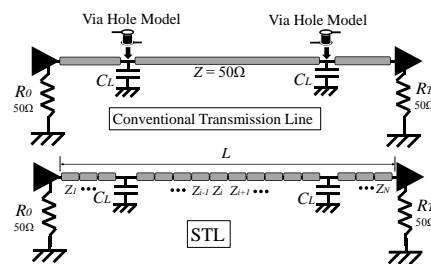
図2 評価対象とした伝送系
