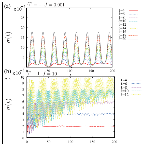
図5：正負の電荷間に張られた電気力線の揺らぎ。
