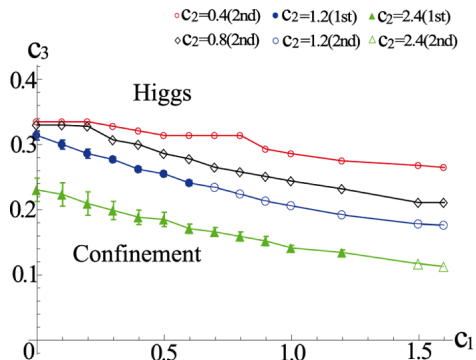
図 2: 3+1次元 U(1)ゲージ・ヒッグスモデルの相構造。ヒッグス相と閉じ込め相がある。
