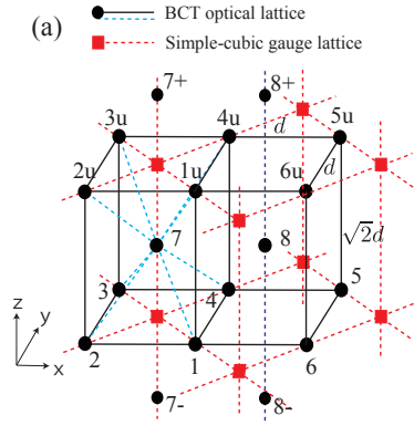
図 1: 光学格子 (黒丸) とゲージ格子 (四角)
