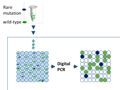
図2 ddPCR
